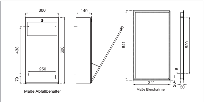
Technische Zeichnung des Abfallbehälters Art. 20-115 und des Blendrahmens für die Einbaumontage.
