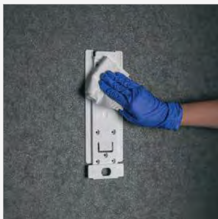
6. Vor der Wiederanbringung des Spenders sollte die montierte Rückwand mit einem in Desinfektionsmittel getauchten Tuch gesäubert werden.
