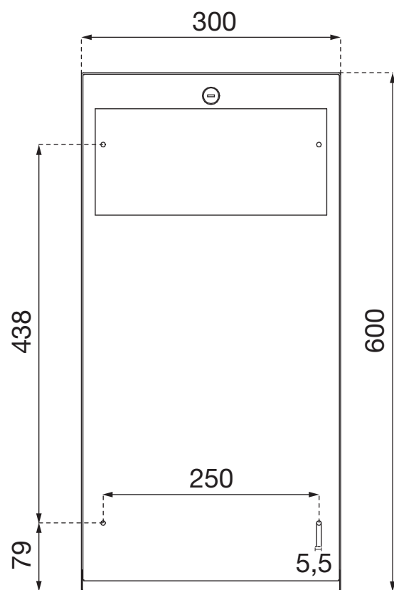
Maße Abfallbehälter
