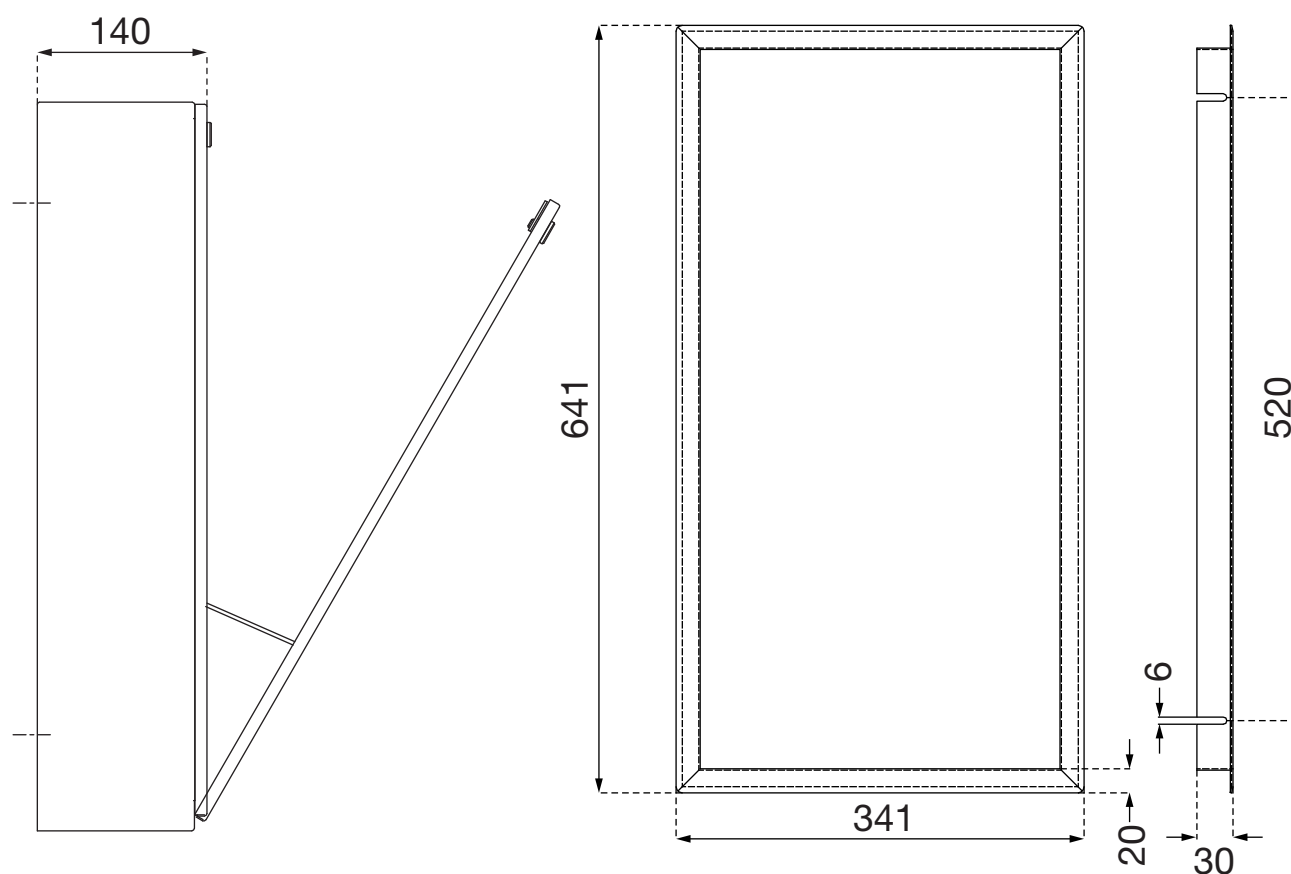
Maße Blendrahmen
