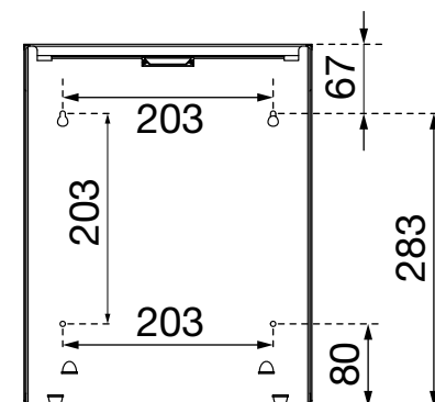
Rückansicht / Bohrbild
