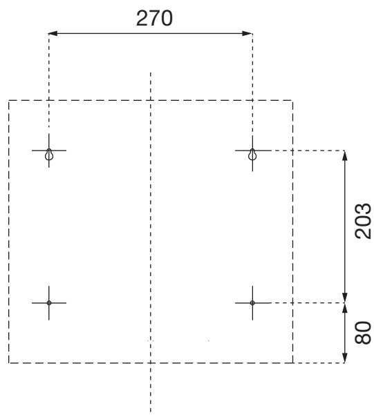
Bohrbild
