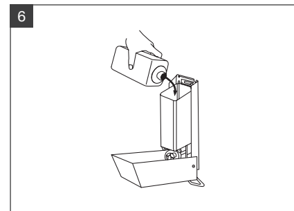
Behälter mit geeignetem Medium auffüllen und Deckel schließen. Fill container with adequate medium and close lid.
