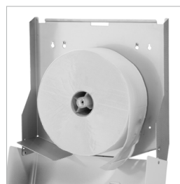
WC-Grossrollenspender für 1 Großrolle, zum Nachfüllen geöffnet
