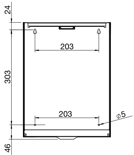
Bohrbild
