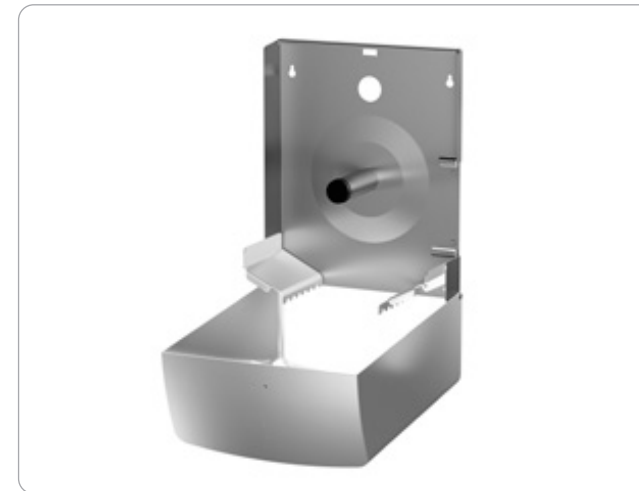
Haushaltsrollen-Adapter entnehmen, um Haushaltsrollenspender zum Großrollenspender umzubauen.
