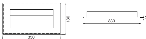
Frontblende
