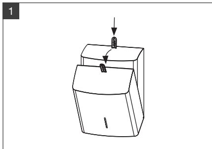
Gehäuse öffnen. Open the unit.
