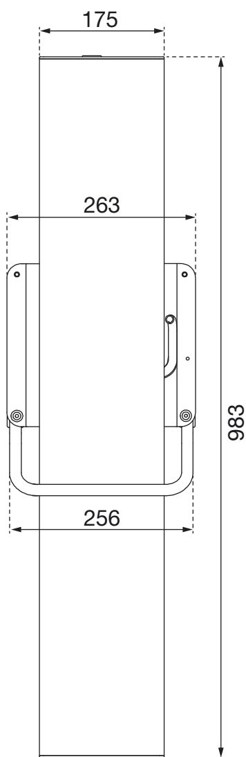
Draufsicht
