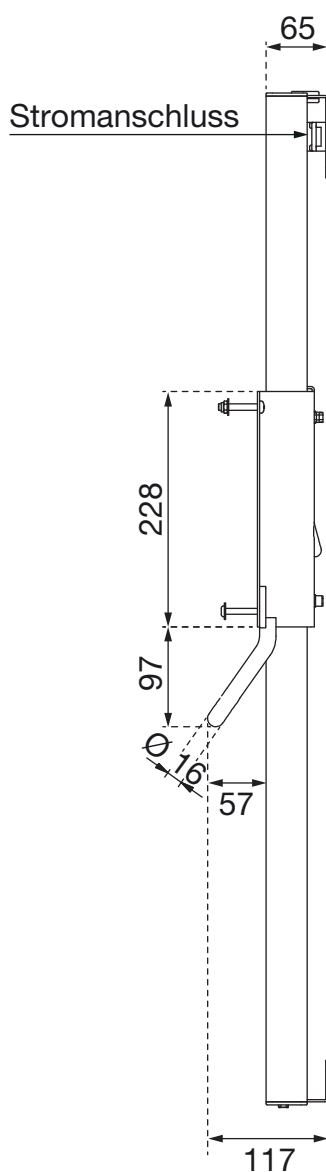
Seitenansicht
