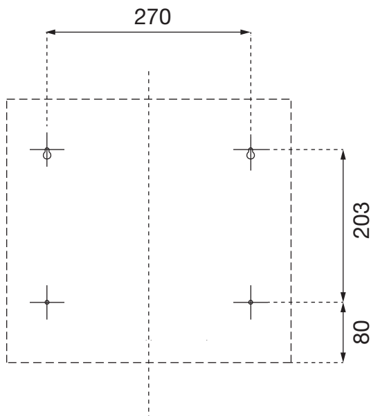
Bohrbild
